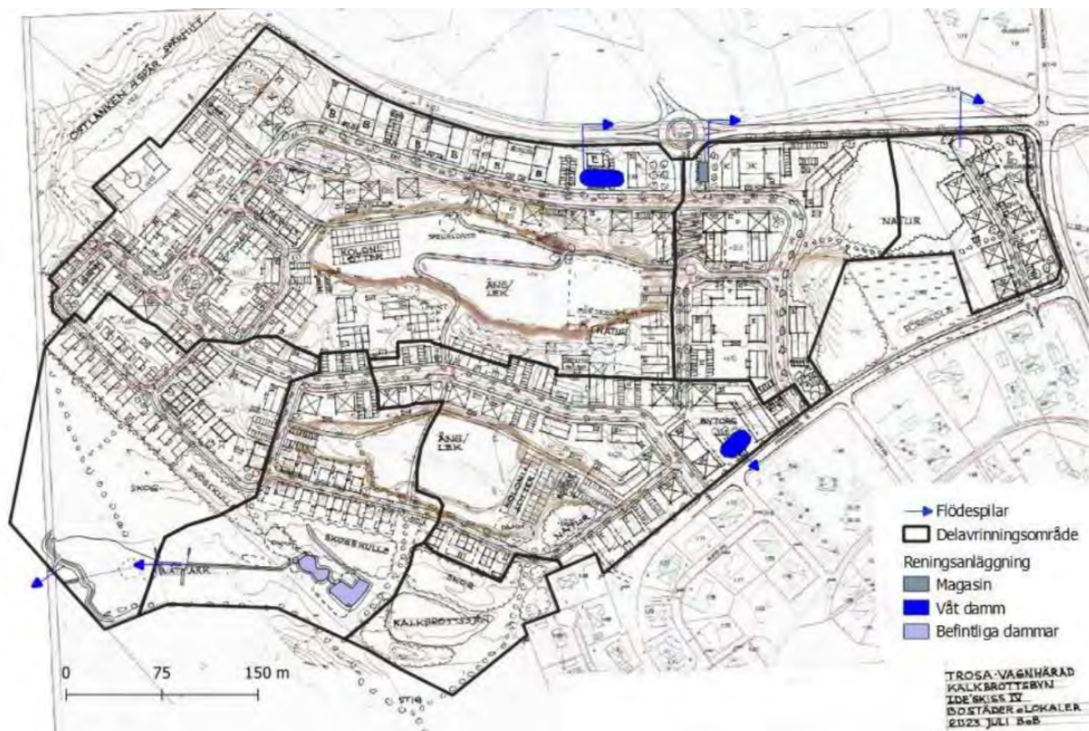
Översiktsbild över reningsanläggningar, ur genomförd dagvattenutredning.
